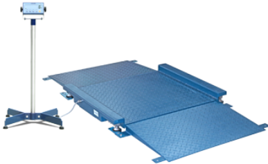
Įrengimo pavyzdys su DFWL indikatoriumi ir CSP38 stulpeliu
